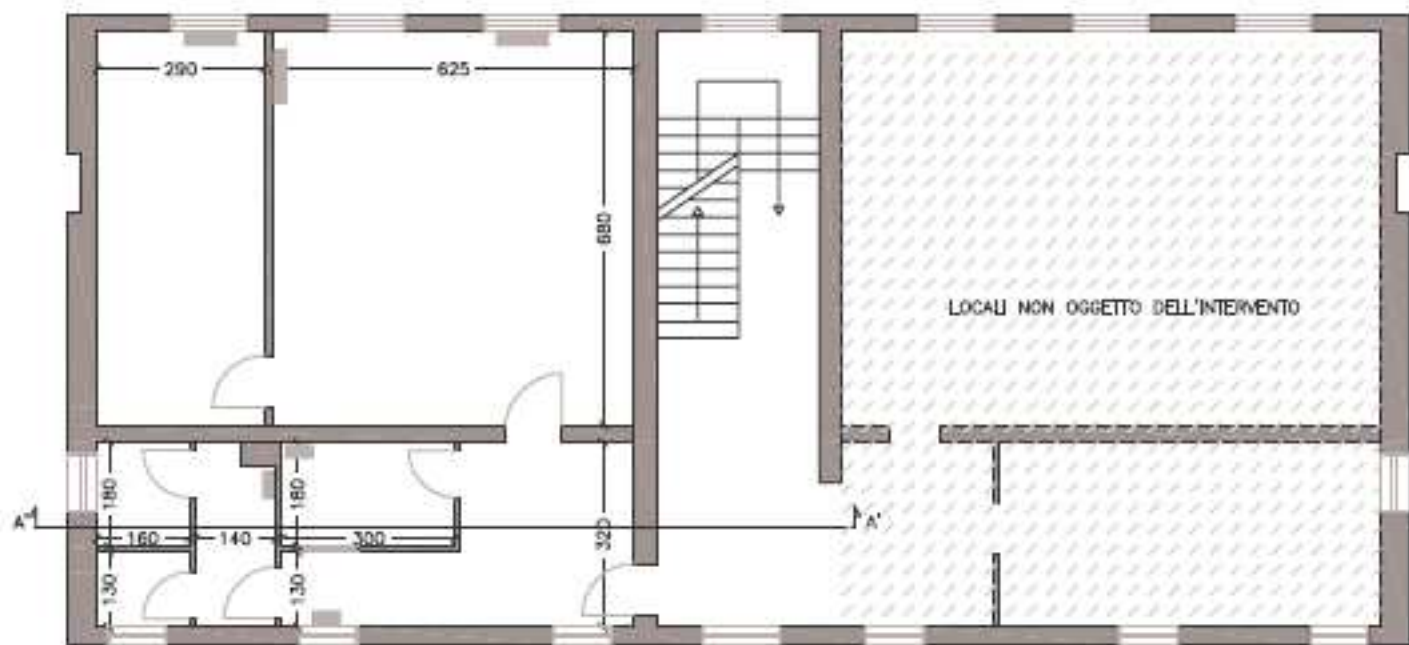
Planimetria piano primo
